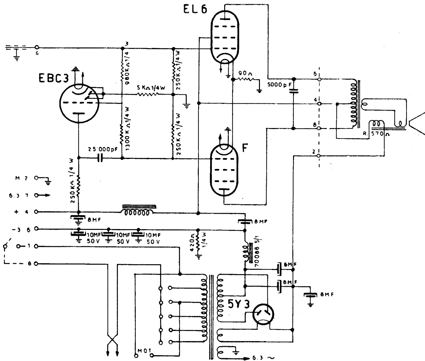
SAVIGLIANO - Mod. OS 710 - Amplificatore finale in controfase e alimentatore anodico. Parte AF/MF stesso circuito e telaio del mod. OS 51. Potenza d'uscita 10 W.
